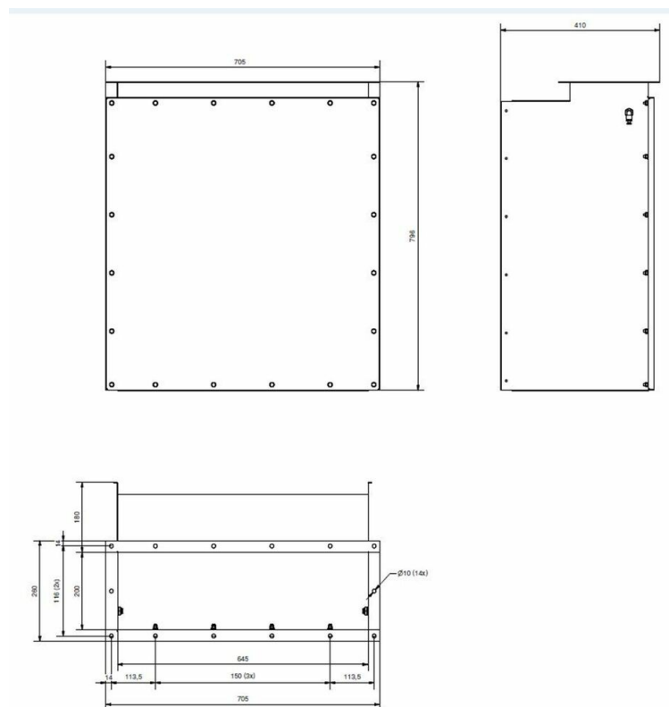
出口接头 OSF 1000FC / OMF 2000FC - HEPA 610x610x292mm
